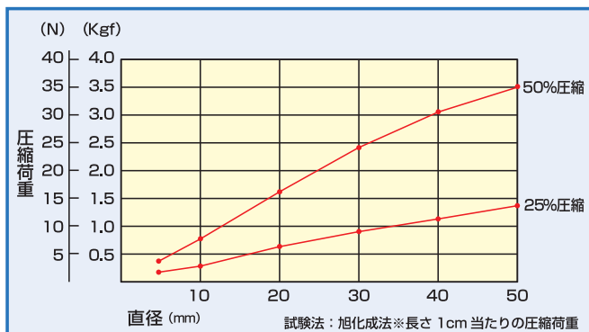
圧縮強度
